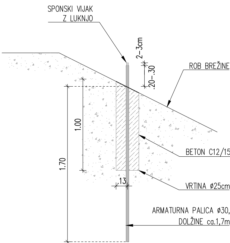
DETAJL MERSKE TOČKE NA RAŠČENEM TERENU Merilo 1:50
